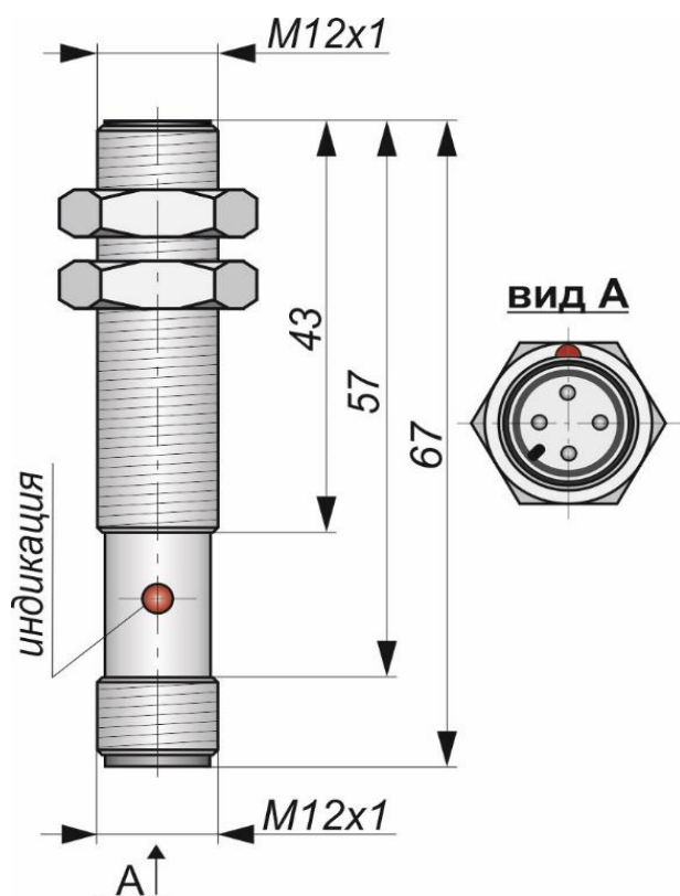
Габаритный чертеж
